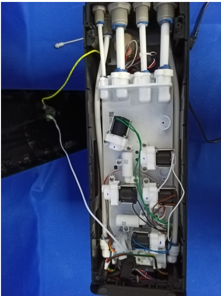
内部结构
